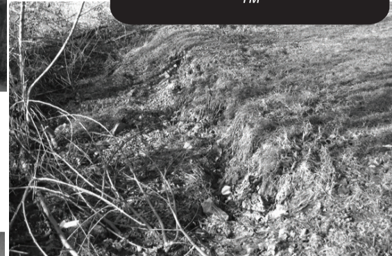
Свлагането на земната маса на места достига до 1м
